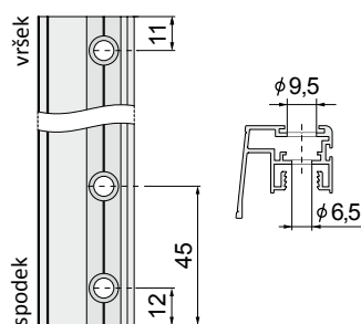
Vrtání otvorů do profilu
