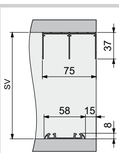
Montáž kolejnic
